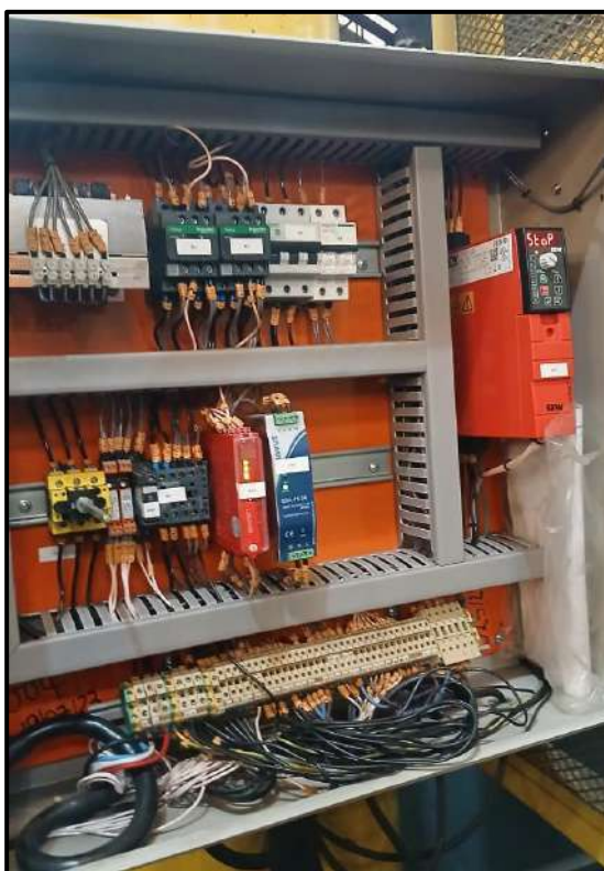
Figura 506: Painel elétrico do braço
