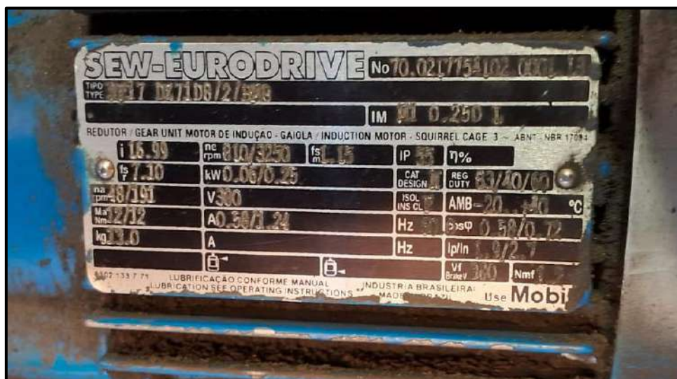
Figura 498: Plaqueta de identificação do motorreductor
