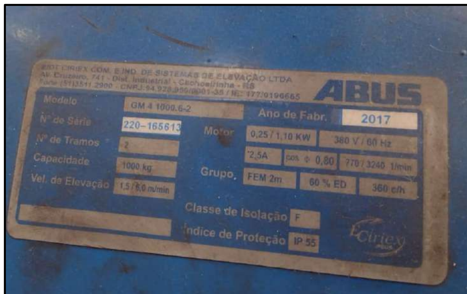
Figura 43: Plaqueta de identificação do motor do trolley
