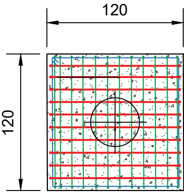
PLANTA BAIXA - ESC 1:25
