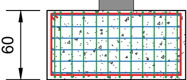
CORTE - ESC 1:25
